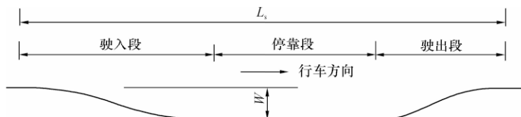
图 5.4.3-4 港湾式停靠站 L_s —港湾长度; W —车道最小宽度
