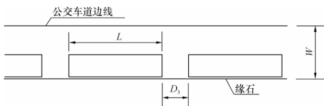
图 5.4.3-3 有超车道不能单独驶入驶出的直列式停靠站 L —公共汽(电)车长度; D_3 —车位间距; W —车道最小宽度
