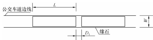
图 5.4.3-1 无超车道直列式停靠站
