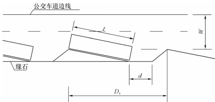
图 5.4.3-5 锯齿式停靠站
