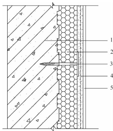
图 6.3.1 EPS 板现浇混凝土外保温系统
