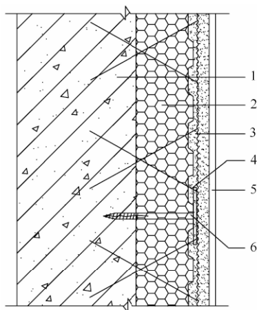
图 6.4.1 EPS 钢丝网架板现浇混凝土外保温系统
