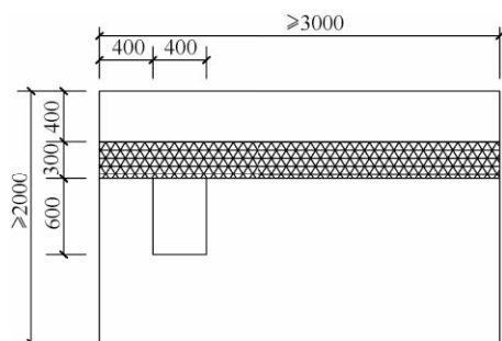
图 A.2.1-2 带防火隔离带试验墙板 (mm)
