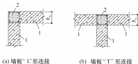
图 6.2.4-3 墙板混凝土构造柱连接
