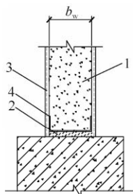
图 6.2.2-2 墙板与基础胶粘剂连接
