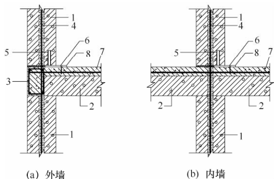
图 6.2.5-2 蒸压加气混凝土墙板与楼板连接
