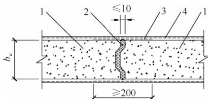
图 6.2.3-2 墙板胶粘剂连接
