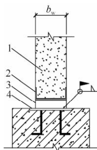
图 6.2.2-1 墙板与基础焊接连接
