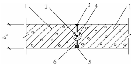
图 6.2.3-3 蒸压加气混凝土墙板连接
