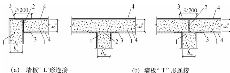
图 6.2.4-2 纵横墙胶粘剂连接
