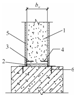
图 6.2.2-3 墙板与基础自攻螺钉连接
