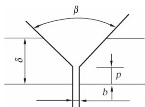
图 A. 2. 2 焊接的坡口形式和对边示意
